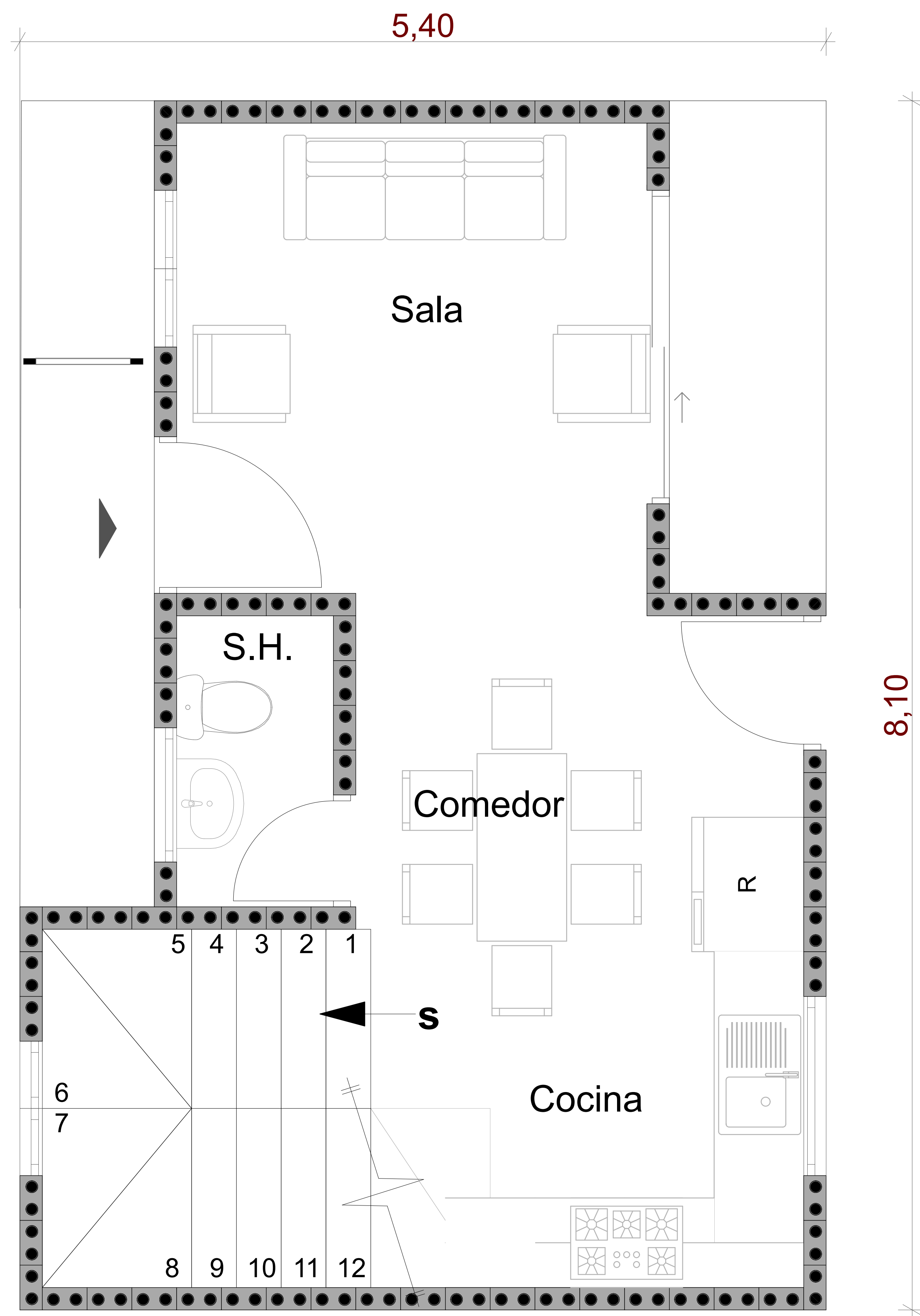
PLANTA BAJA
