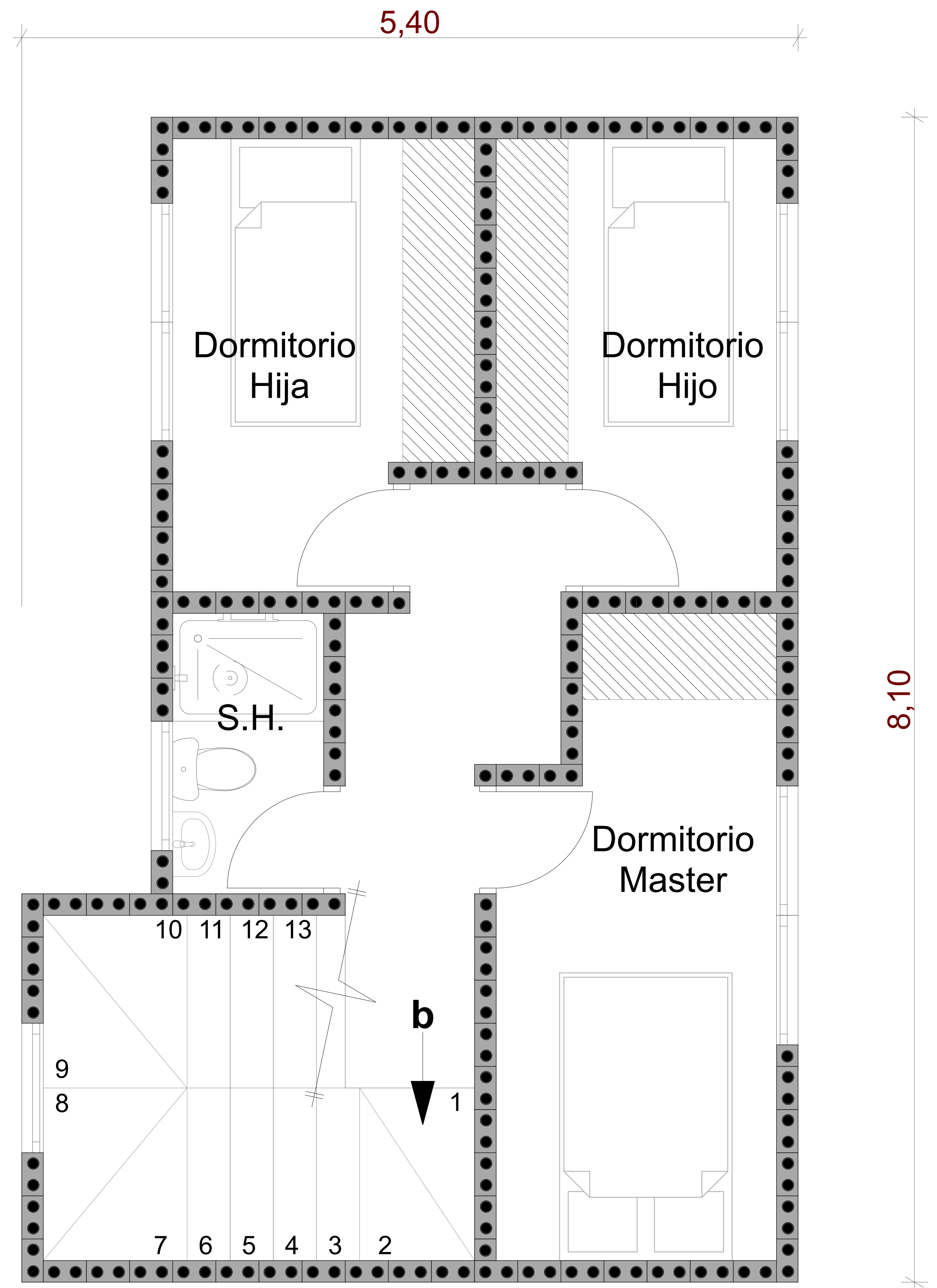
PLANTA ALTA
